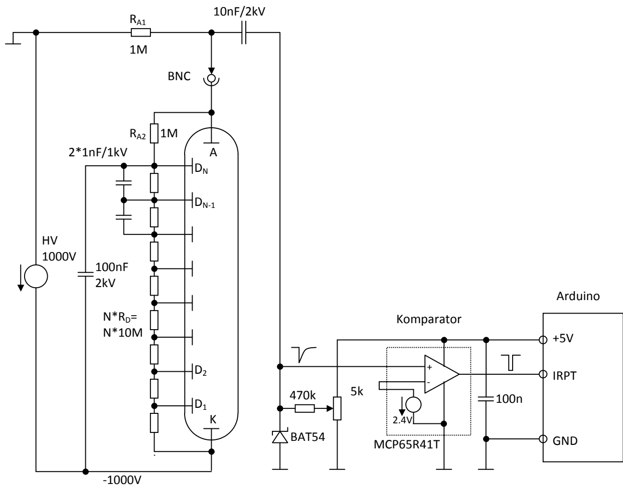
PMT-zu-Arduino Adapter für negative Hochspannungsversorgung (Update16.2.2016)
